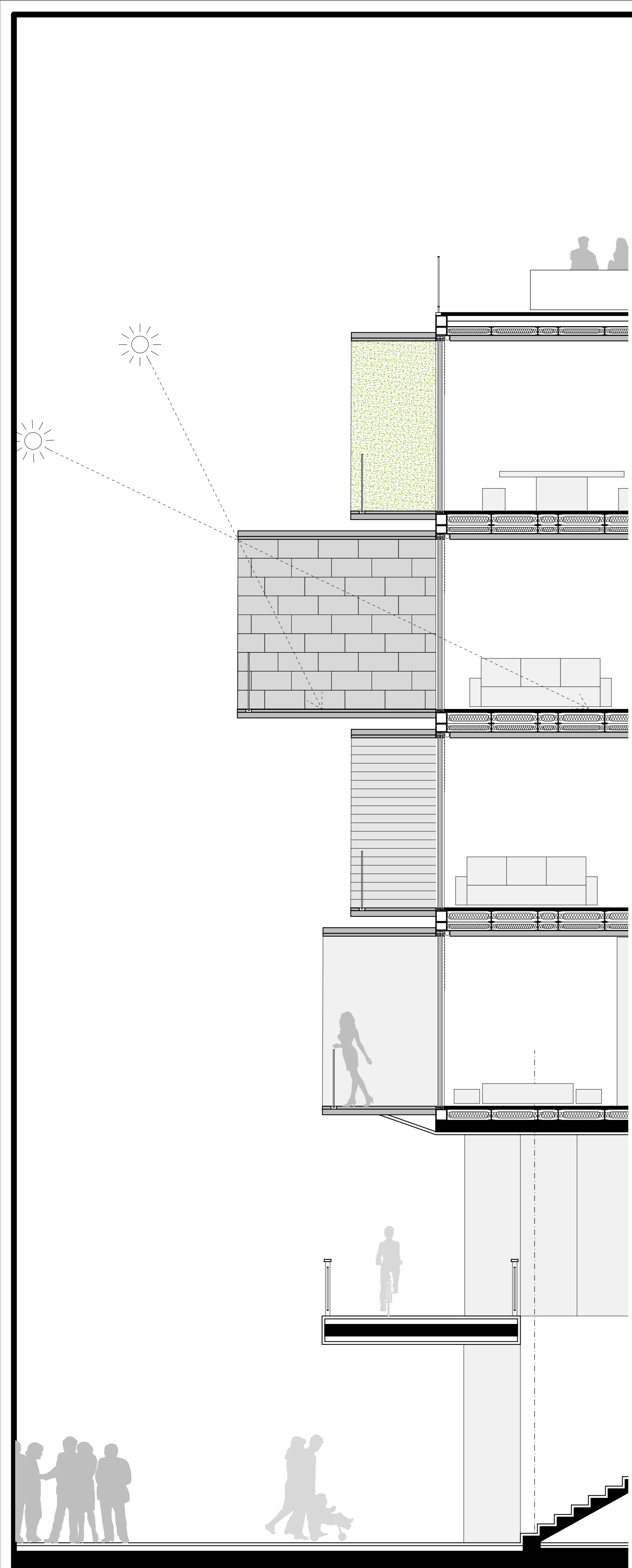
SEZIONE DEGLI ALLOGGI SUL PORTO CANALE SCALA 1:50
